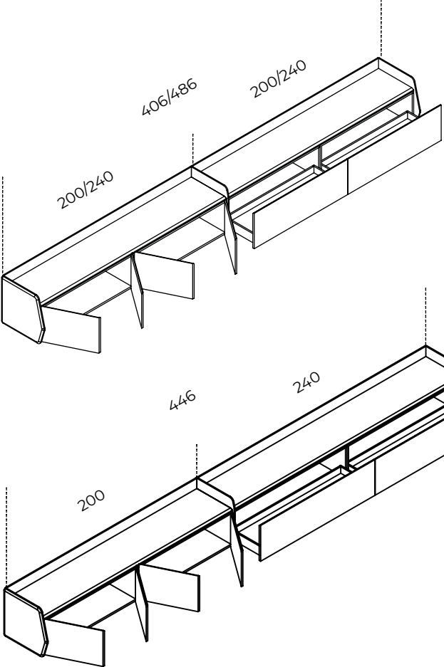
Versione AACC (ante/cassettoni) Version AACC (doors/large drawers)
